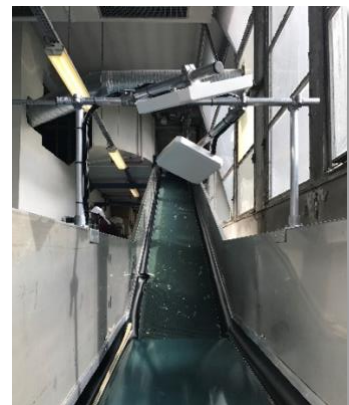
- Convoyeur RFID -
